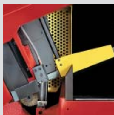
pattino regolabile (solo 330) adjustable blade guide (only 330)
